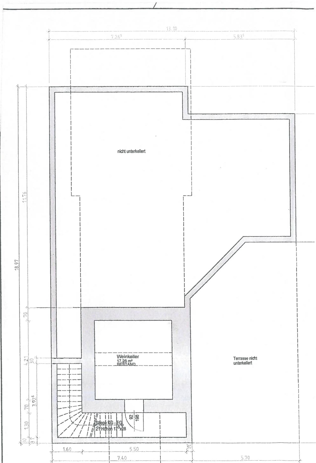
Grundriss KG
